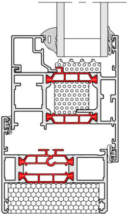
58BW CASEMENT HI JAMB
