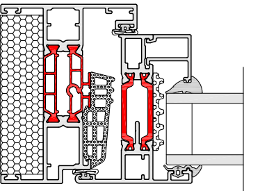
58BW ST FLUSH HI JAMB SECTION 1
